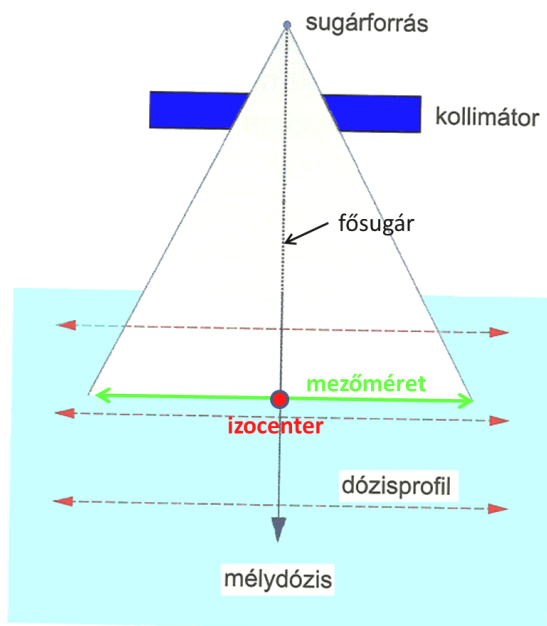
13.1. ábra. A sugárnyaláb jellemző paraméterei.
