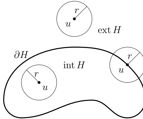
10.4. ábra. Halmaz belső, külső és határpontja
