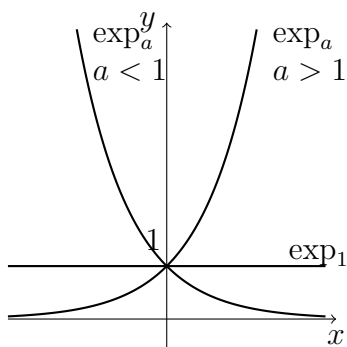
2.8. ábra. Különböző alapú exponenciális függvények
