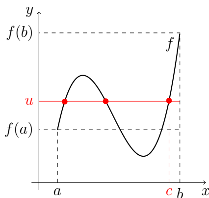
4.10. ábra. Bolzano–Darboux-tétel
