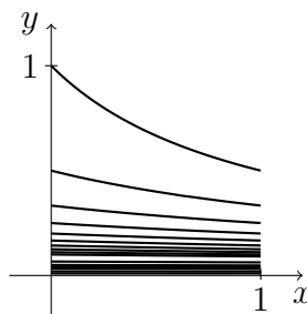
8.5. ábra. f_n(x) = \frac{1}{x+n} konvergenciája
