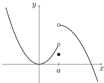
4.7. ábra. Ugráshely
