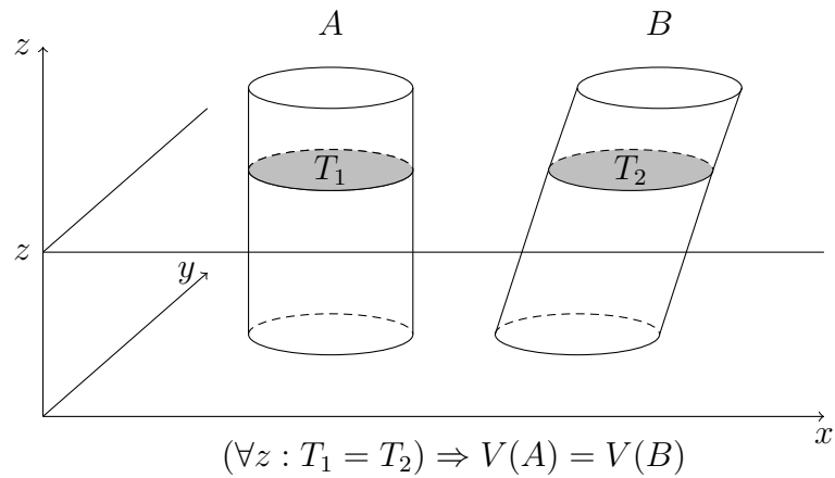
13.4. ábra. Cavalieri-elv
