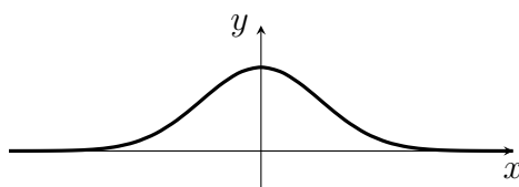
7.7. ábra. Az f(x) = e^{-x^2} függvény grafikonja („haranggörbe”)
