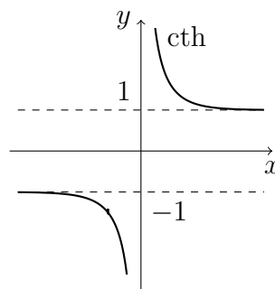
2.24. ábra. A \operatorname{cth} függvény
