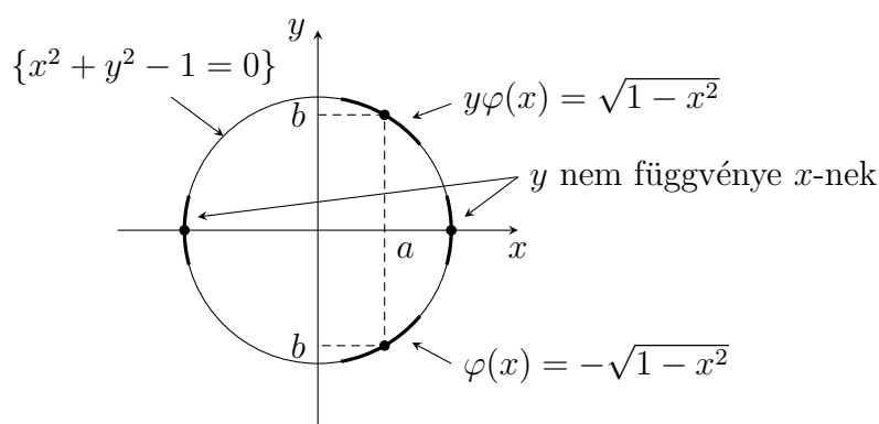
17.1. ábra. Egyváltozós implicitfüggvény-tétel példa
