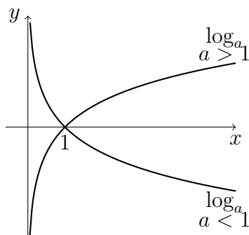
2.10. ábra. Különböző alapú logaritmusfüggvények
