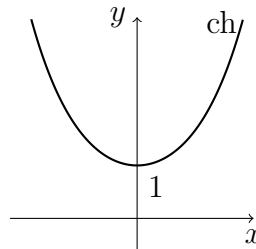
2.22. ábra. A \text{ch} függvény
