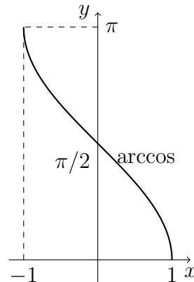
2.18. ábra. Az arccos függvény
