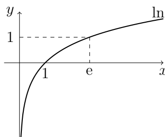
2.11. ábra. Természetes alapú logaritmusfüggvény
