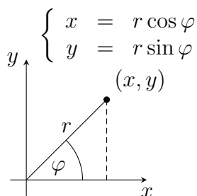
16.3. ábra. Polárkoordináták
