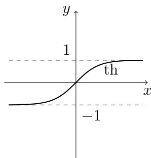
2.23. ábra. A \operatorname{th} függvény
