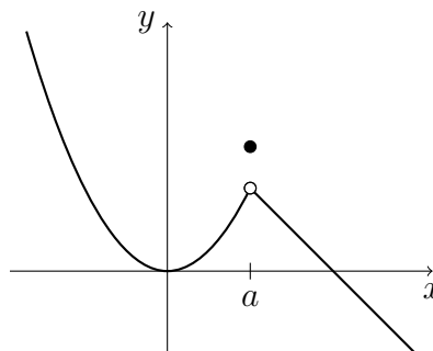
4.8. ábra. megszüntethető szakadási hely
