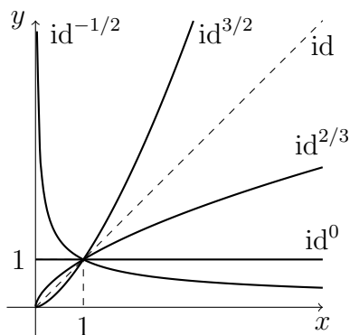
2.7. ábra. Néhány hatványfüggvény
