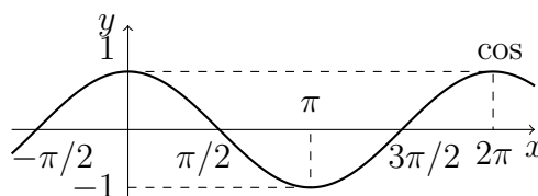
2.14. ábra. A \cos függvény
