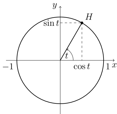
18.1. ábra. A \gamma : [0, 2\pi] \rightarrow \mathbb{R}^2 , \gamma(t) = (\cos t, \sin t) síkgörbe értékkészlete
