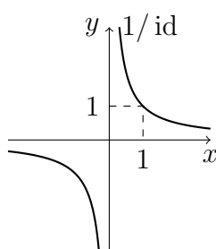
2.4. ábra. Az 1/id függvény
