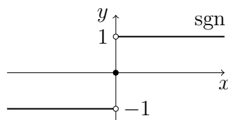
2.30. ábra. Az előjelfüggvény
