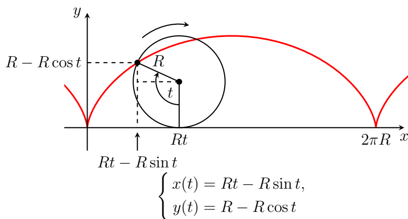
18.2. ábra. Ciklois
