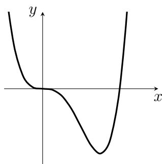
6.10. ábra. Az f(x) = x^4 - 2x^3 függvény grafikonja
