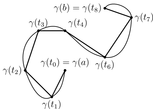
18.3. ábra. Beírt töröttvonal
