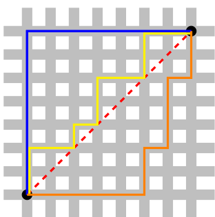
10.1. ábra. „Manhattan-távolság”
