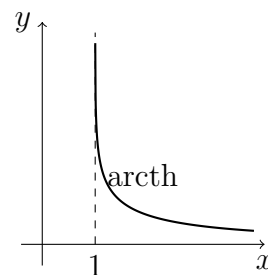
2.28. ábra. Az archth függvény
