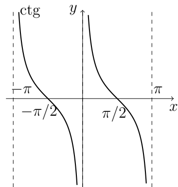
2.16. ábra. A ctg függvény
