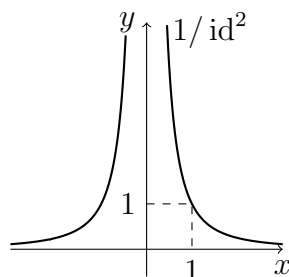
2.5. ábra. Az 1/id^2 függvény
