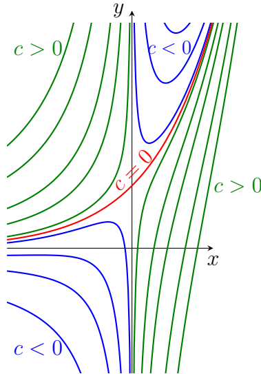
14.3. ábra. Az y'(x) + \frac{y(x)}{x} = \frac{x+1}{x} e^x egyenlet megoldásai: e^x + \frac{c}{x}
