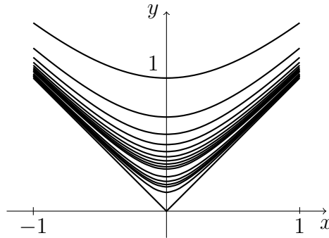
8.9. ábra. f_n(x) = \sqrt{x^2 + \frac{1}{n}} , n \in \mathbb{N} konvergenciája
