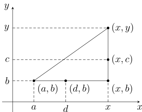
15.5. ábra. Folytonos parciális deriváltak és differenciálhatóság, bizonyítás
