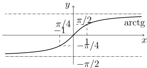
2.19. ábra. Az \text{arctg} függvény
