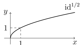
2.6. ábra. Az id^{1/2} függvény
