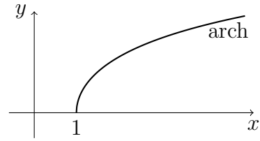
2.26. ábra. Az arch függvény
