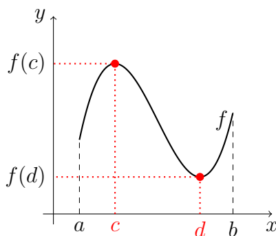
4.11. ábra. Weierstrass-tétel
