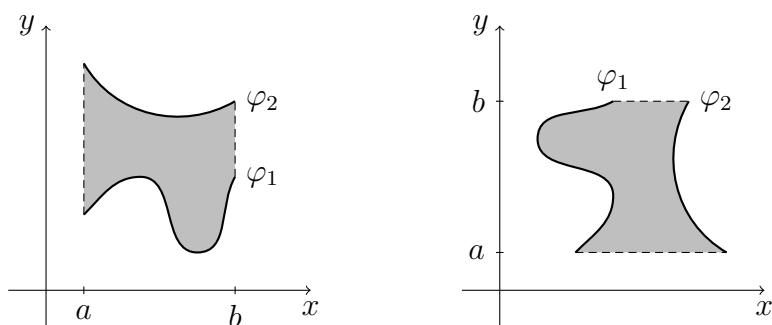
13.3. ábra. Normáltartományok
