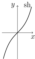
2.21. ábra. Az \text{sh} függvény
