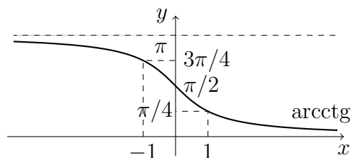
2.20. ábra. Az \text{arcctg} függvény
